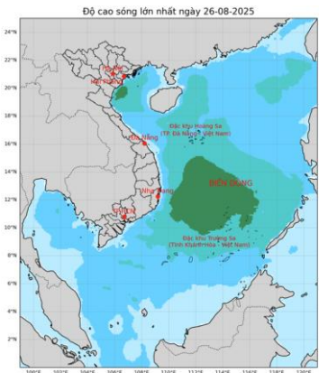
Hình 2. Bản đồ dự báo độ cao sóng
